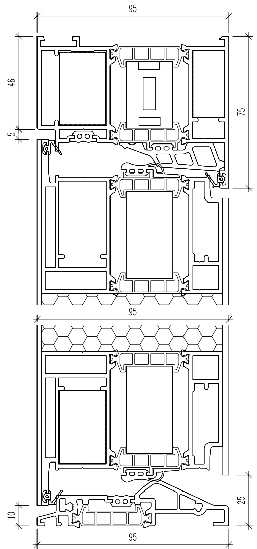
VERTIKALSCHNITT
